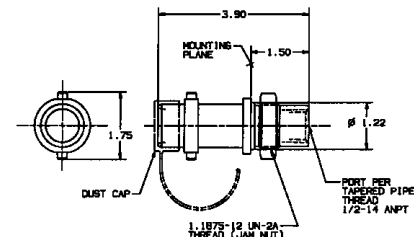
Receptacle 50E721
